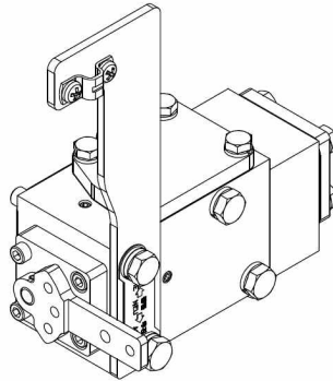
변환밸브그룹
