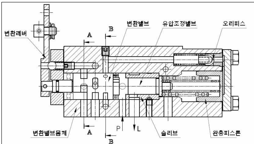
[그림-6 변환밸브그룹]
