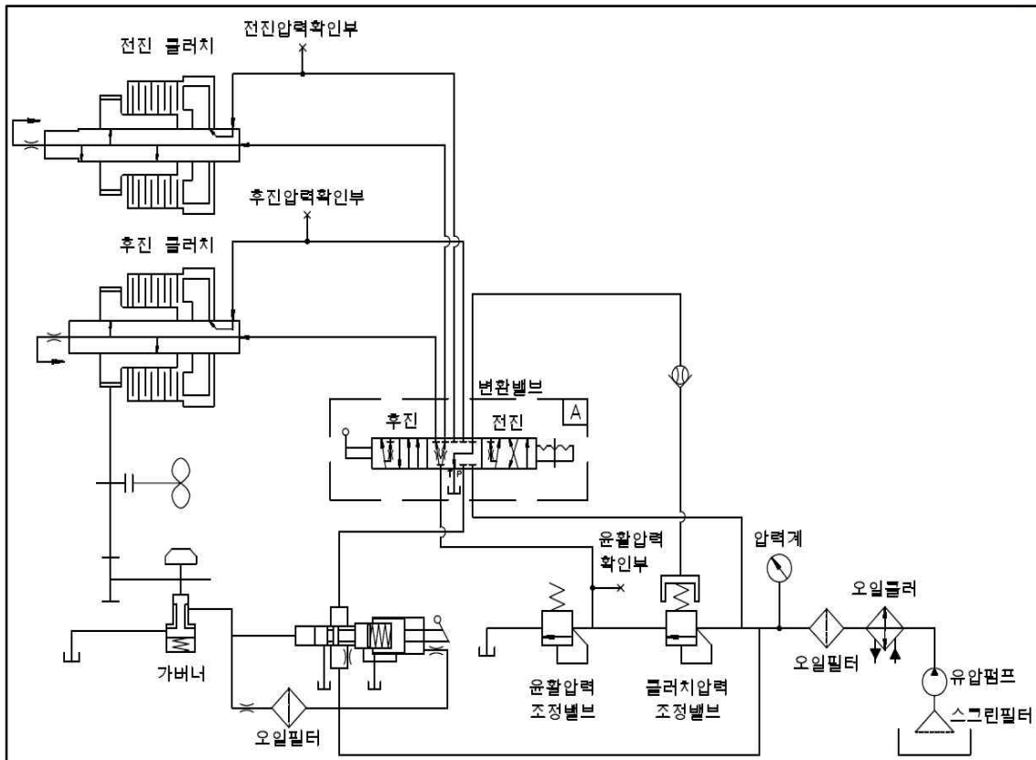
[그림-4.2 유압회로도] - D 트롤링 펌프_옵션
