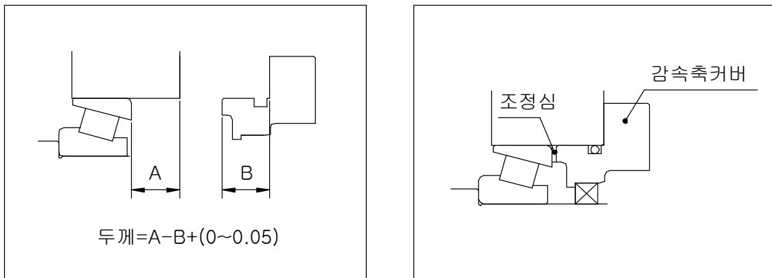
[그림-11] 감속축 심조정
