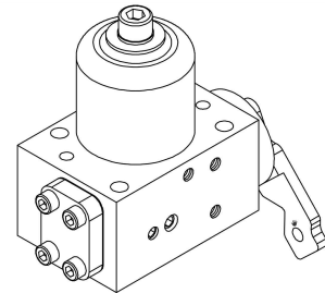
D 트롤링밸브그룹
