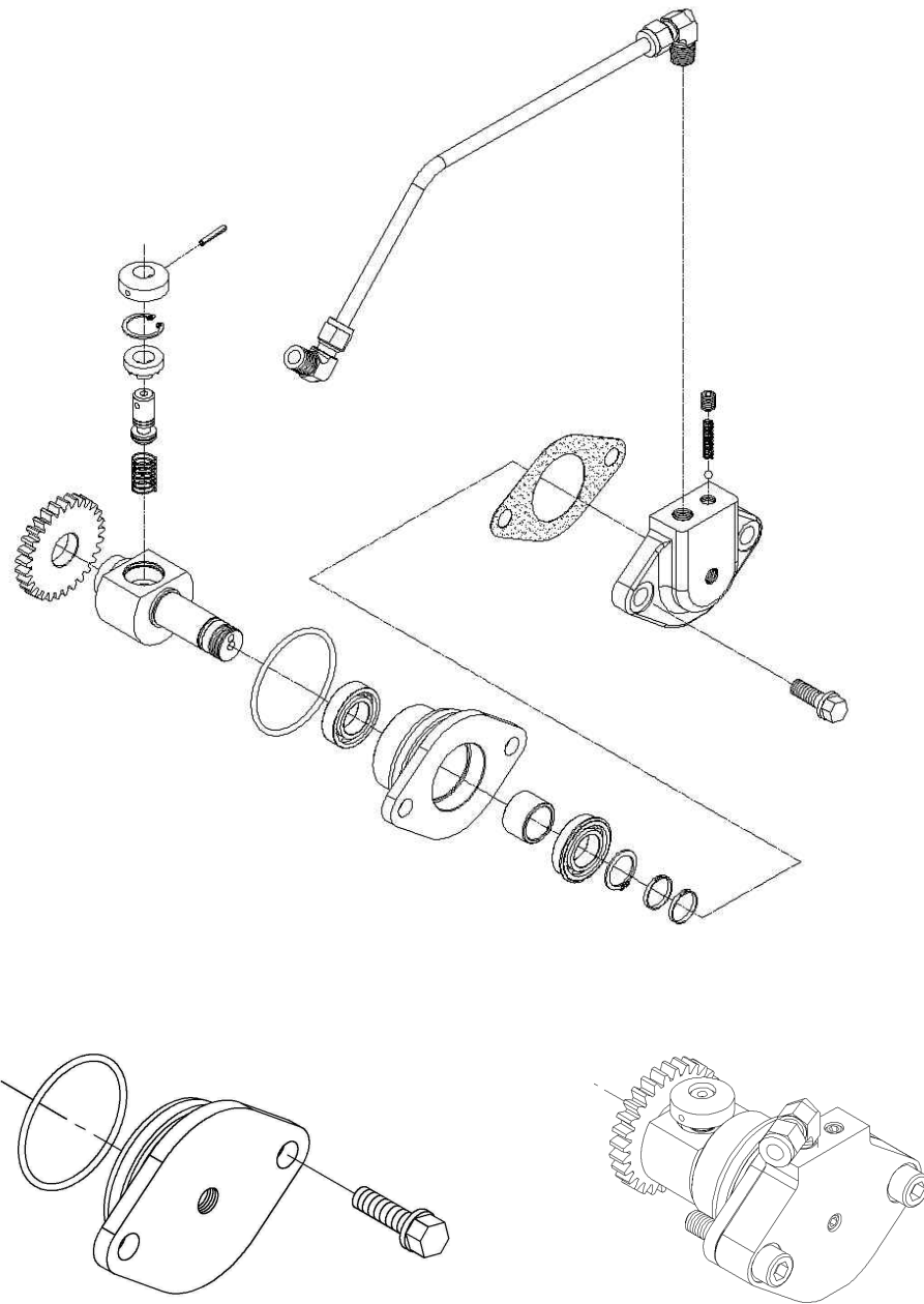
일반변환밸브그룹 + 가버너커버
