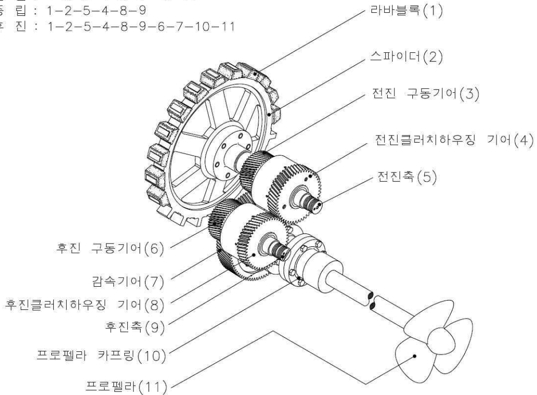
[그림-2 동력전달계통]
